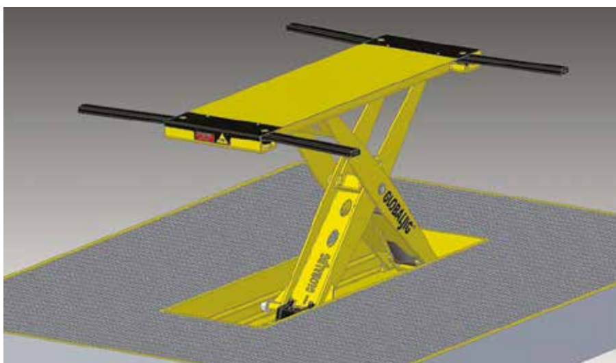
SOLLEVATORI PER ZONE DI PREPARAZIONE
