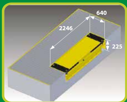
DIMENSIONI DI INCASSO CON SOLLEVATORE CHIUSO
